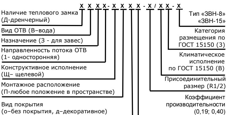
Структура обозначения оросителей по ГОСТ Р 51043-2002
